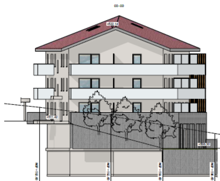
BATIMENT C - FACADE OUEST
